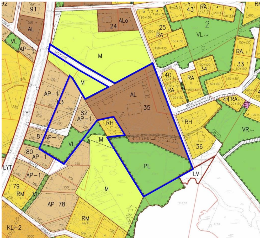
Kuva 6. Ote ajantasa-asetmakaavasta.
