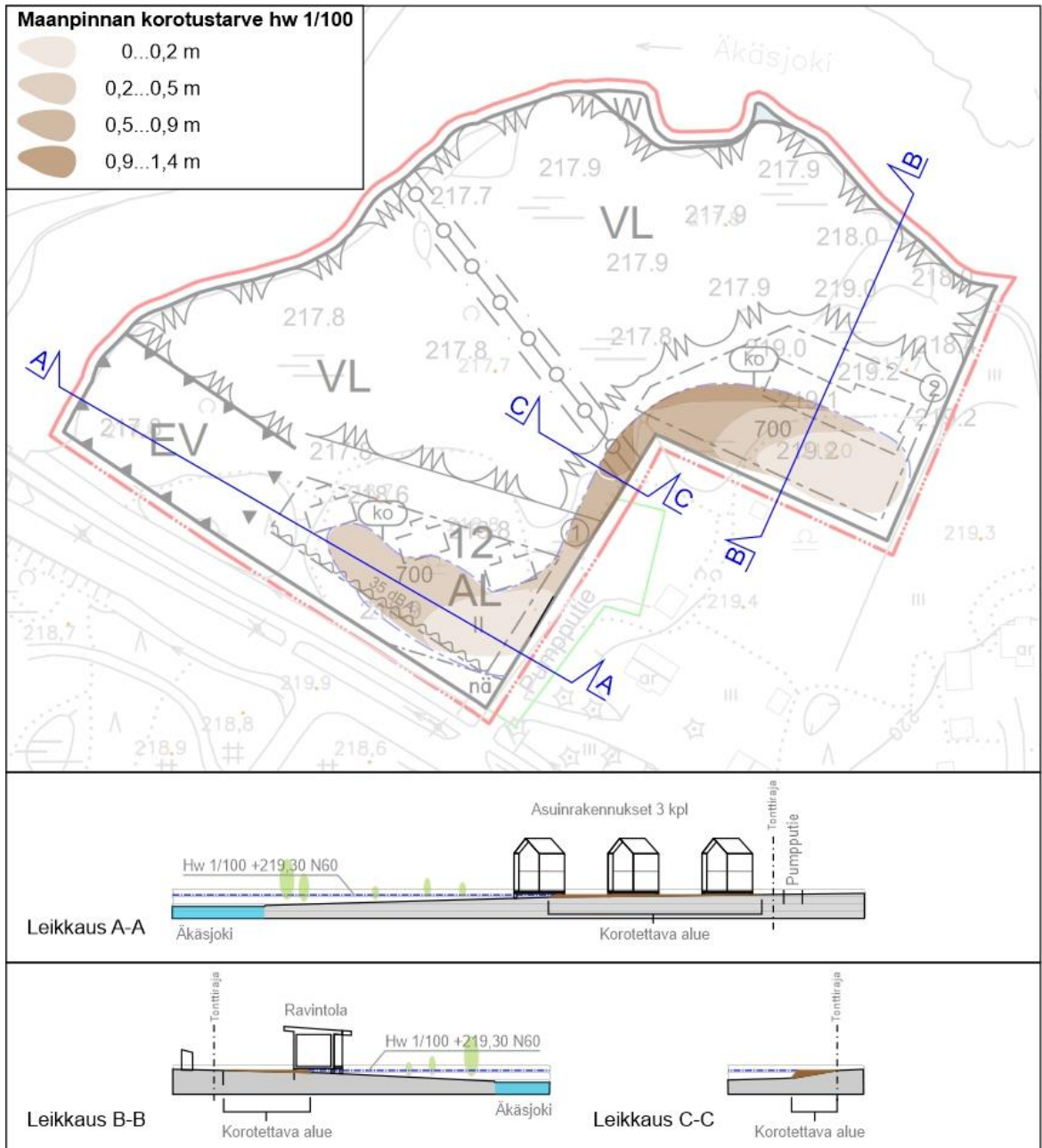
Kuva 22. Maanpinnan korotustarve ja alueleikkaukset A-A, B-B ja C-C.
