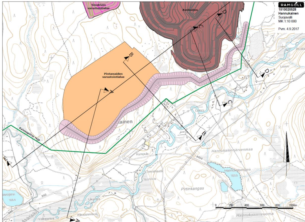
Kuva 5-1 Suojavallin asemapiirros sekä poikkileikkauspaikat. Kartta ja kaikki leikkauspiirrokset ovat suunnitelman liitteenä 3.
